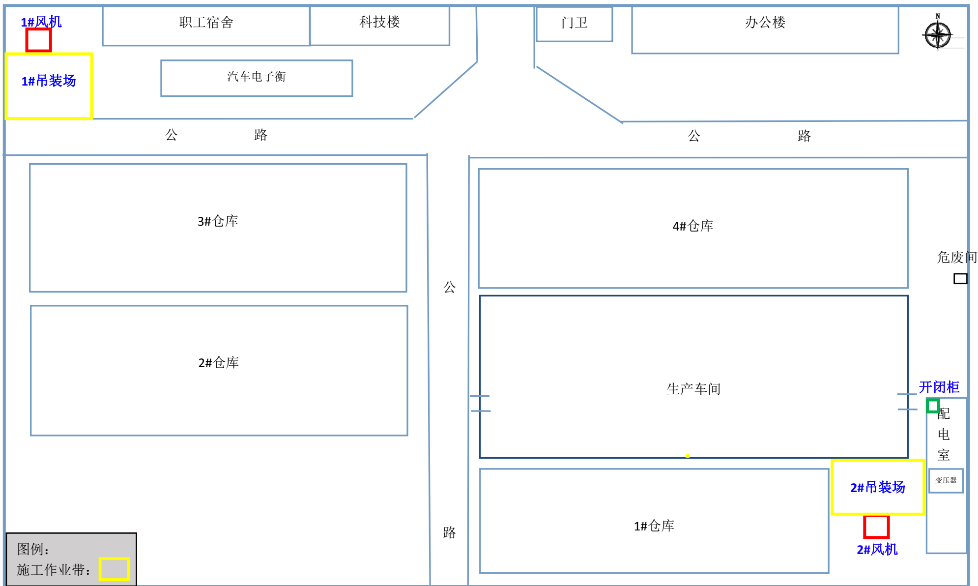
附图3 施工平面布置图
