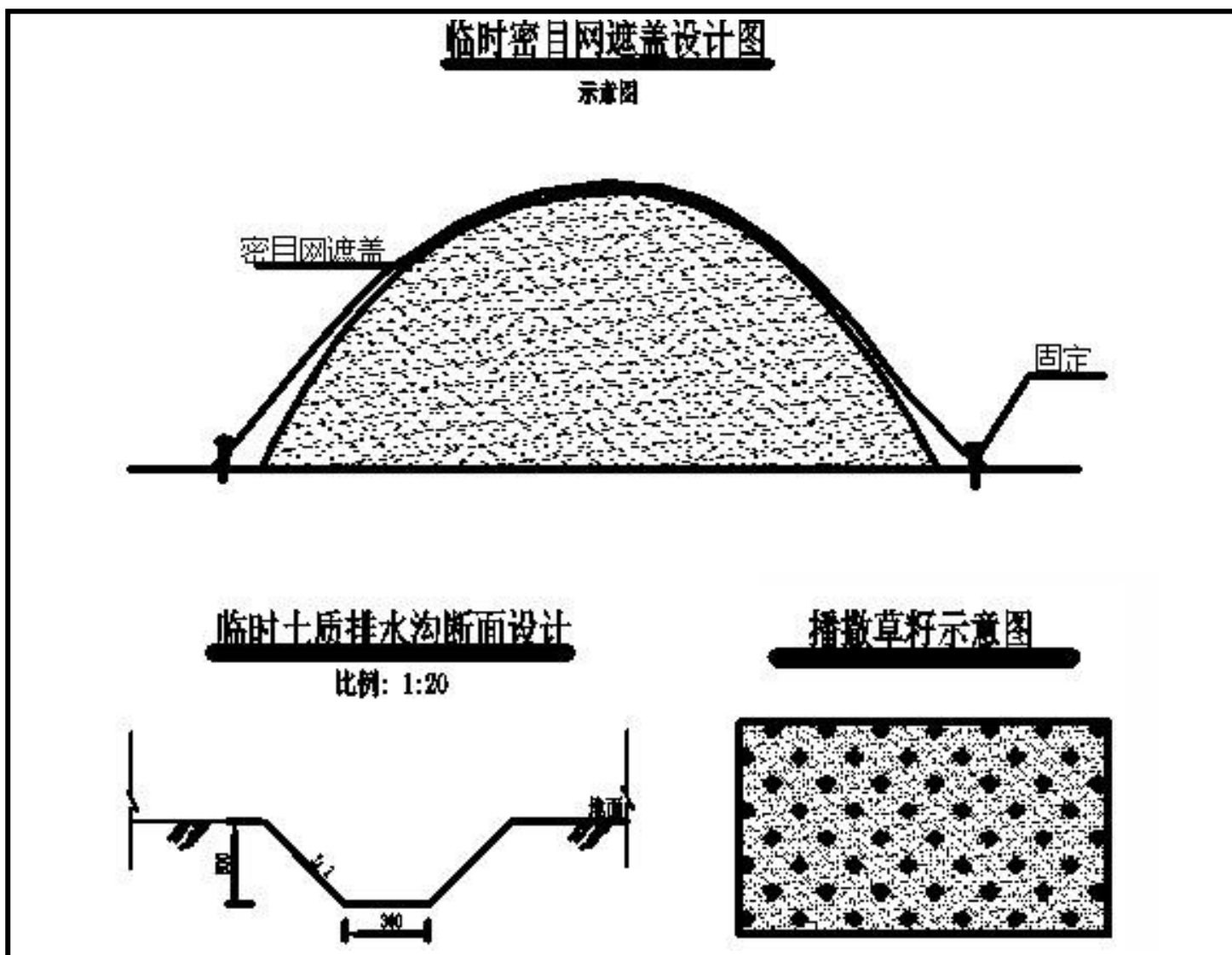
附图 8 项目典型生态保护措施设计示意图
